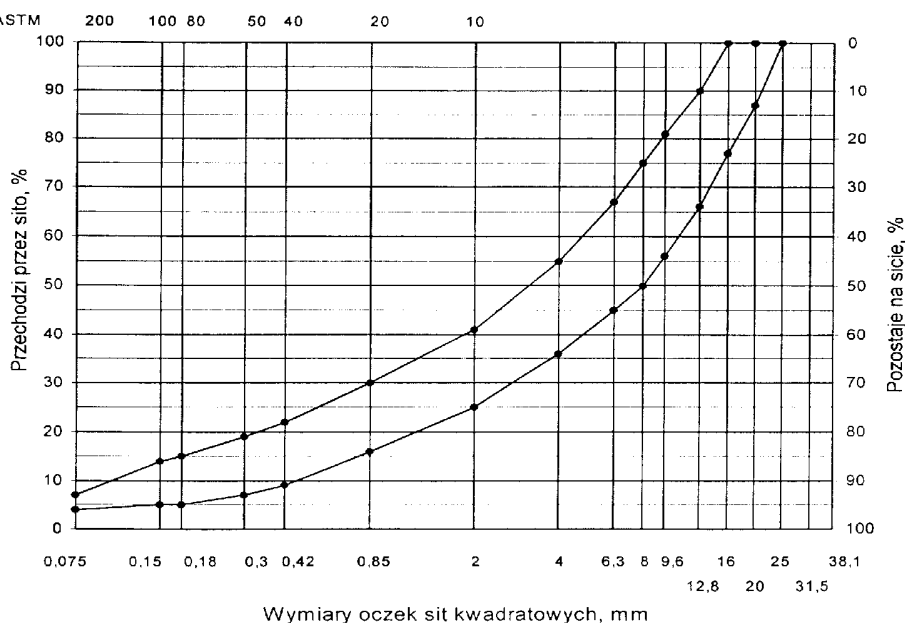
Rys. 4. Krzywe graniczne uziarnienia mieszanki mineralnej BA od 0 do 20 mm do warstwy wiążącej, wyrównawczej i wzmacniającej nawierzchni drogi o obciążeniu ruchem od KR3 do KR6
