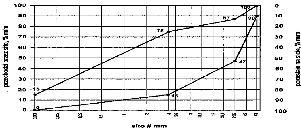
Rys. 1. Krzywe graniczne uziarnienia mieszanki kruszyw 0/63 mm do warstwy mrozochronnej
